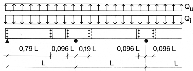
Fig 6 Skarvning av Z-balkar
