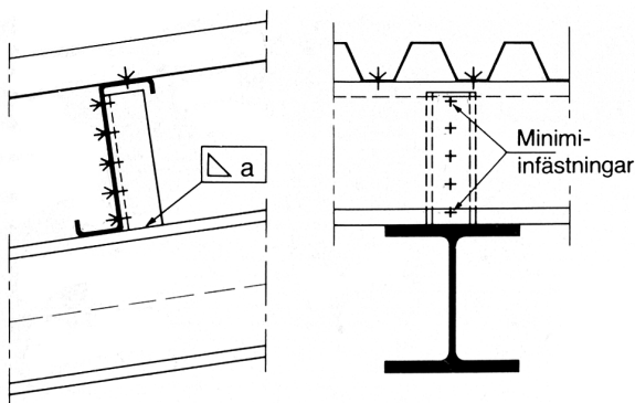
Fig 4 Upplagskonsol i takbalk
